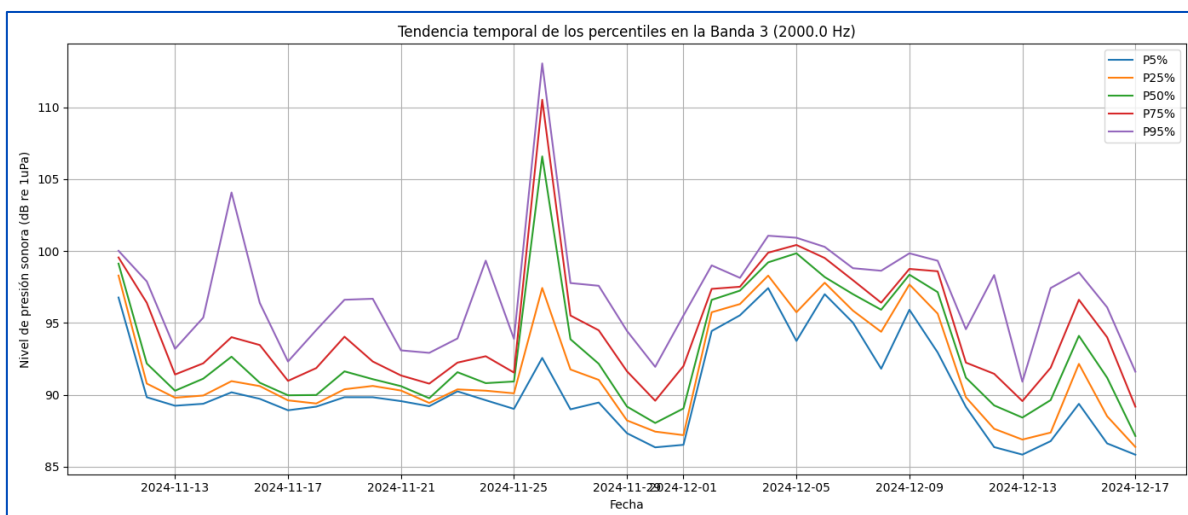
Gráfico 16. Serie temporal de los niveles de SPL en los percentiles 5, 25, 50, 75 y 95, de la banda de 2 KHz, calculados para una ventana temporal de integración de 1 hora. Periodo de invierno.
