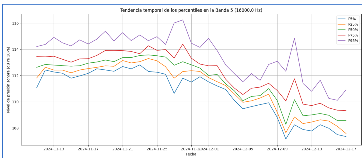
Gráfico 18. Serie temporal de los niveles de SPL en los percentiles 5, 25, 50, 75 y 95, de la banda de 16 KHz, calculados para una ventana temporal de integración de 1 hora. Periodo de invierno.
