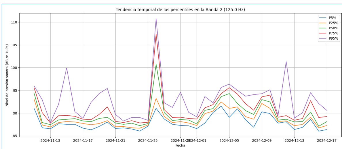
Gráfico 15. Serie temporal de los niveles de SPL en los percentiles 5, 25, 50, 75 y 95, de la banda de 125Hz, calculados para una ventana temporal de integración de 1 hora. Periodo de invierno.
