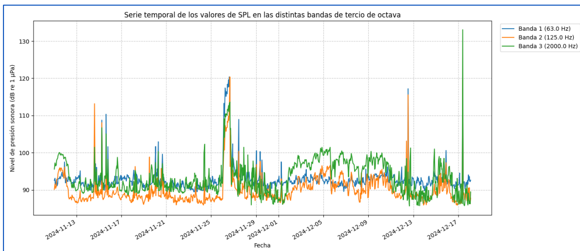
Gráfico 13. Serie temporal de los niveles de presión sonora en las diferentes bandas de tercio de octava, durante el periodo de invierno.
