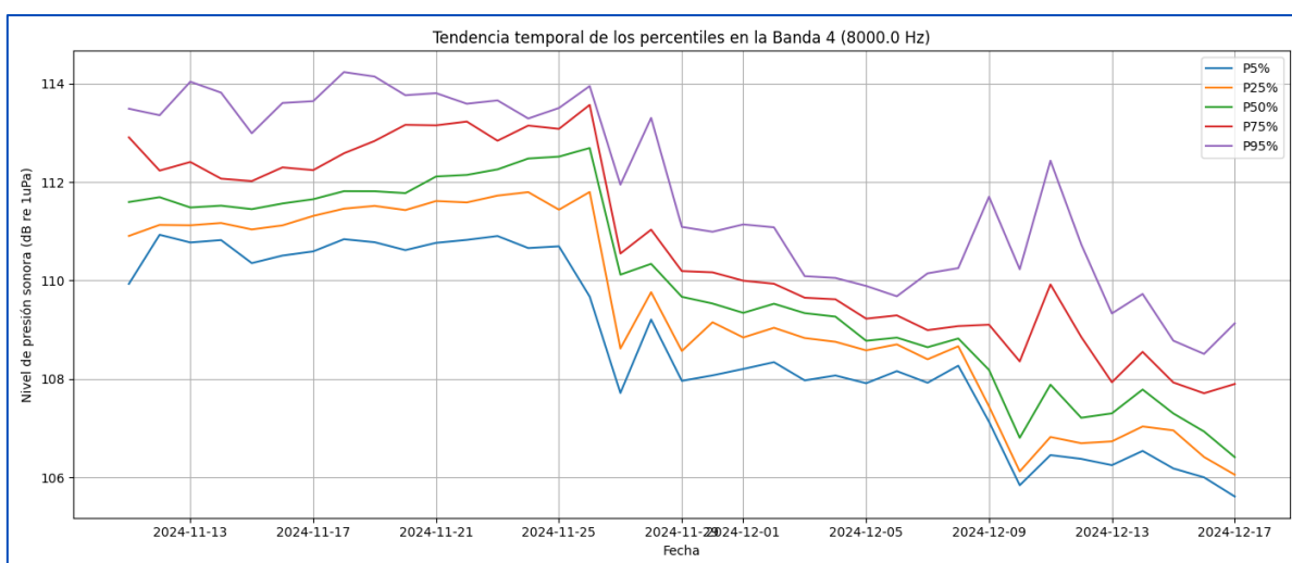
Gráfico 17. Serie temporal de los niveles de SPL en los percentiles 5, 25, 50, 75 y 95, de la banda de 8 KHz, calculados para una ventana temporal de integración de 1 hora. Periodo de invierno.
