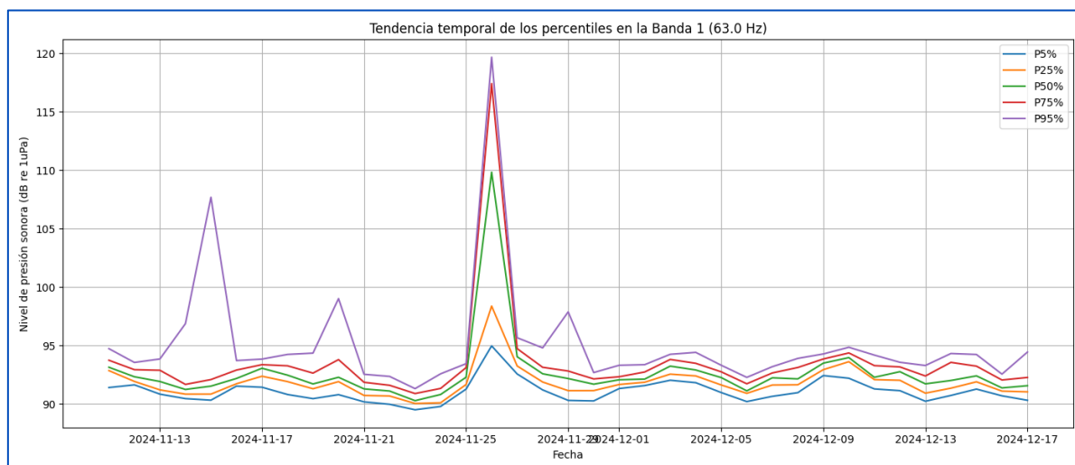
Gráfico 14. Serie temporal de los niveles de SPL en los percentiles 5, 25, 50, 75 y 95, de la banda de 63Hz, calculados para una ventana temporal de integración de 1 hora. Periodo de invierno.
