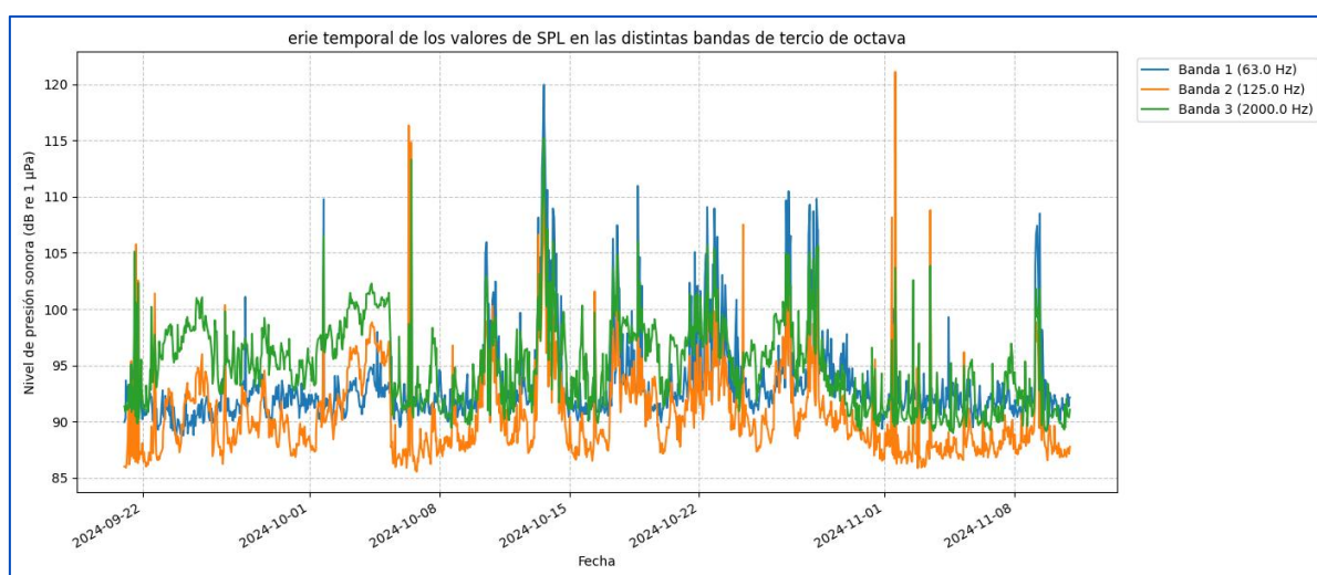
Gráfico 7. Serie temporal de los niveles de presión sonora en las diferentes bandas de tercio de octava, durante el periodo de otoño.
