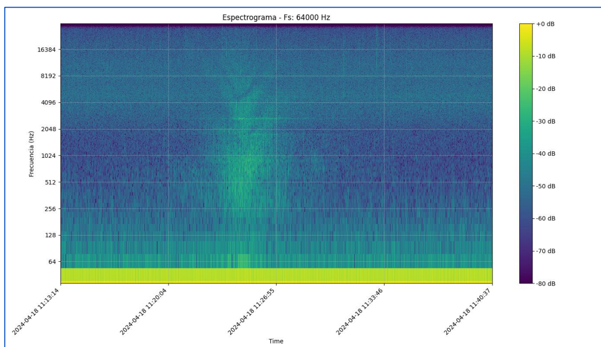
Ilustración 5. Espectrograma donde se muestra un efecto Doppler causado por el paso de una embarcación, con un consecuente aumento del nivel de presión sonora.
